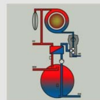
Схема роботи котла Vitodens 333-F, тип WS3C
